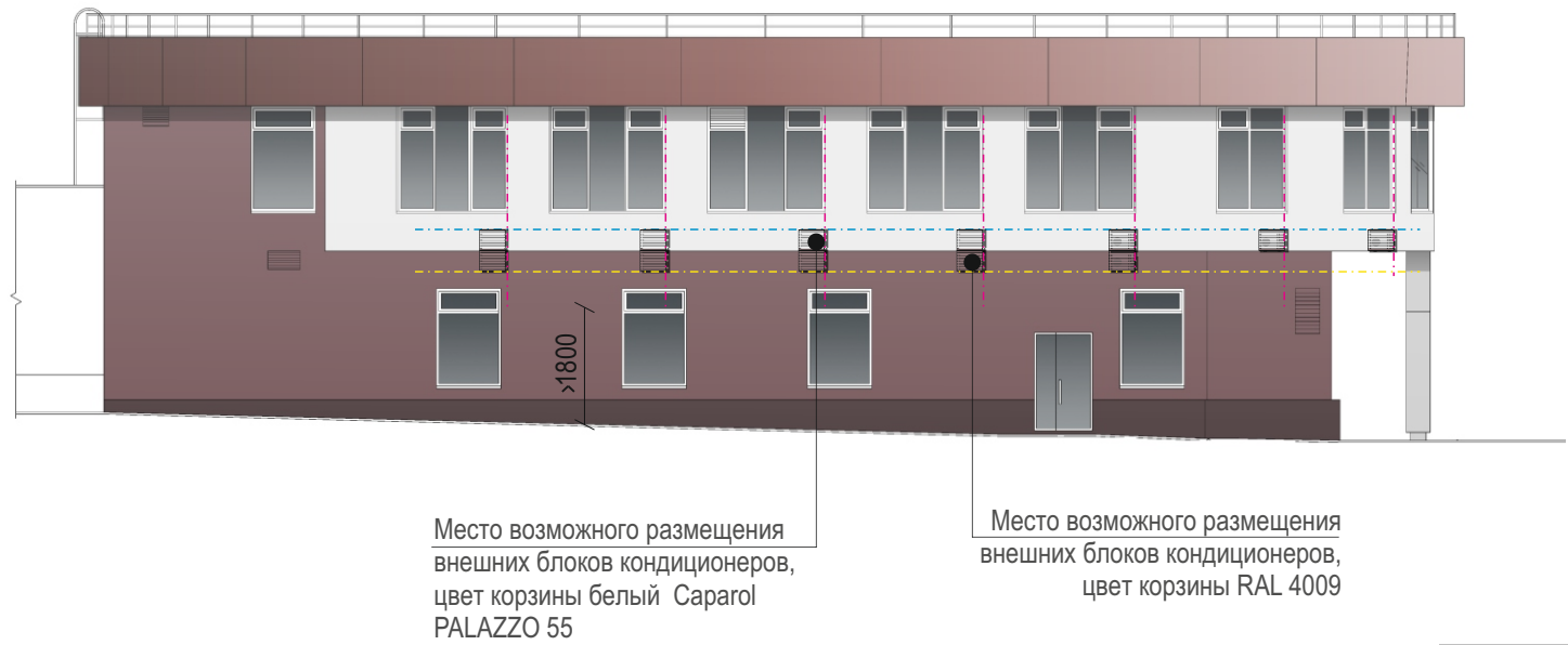
Фрагмент дворового фасада. М 1:200 в
